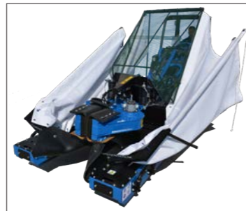
BOOMSCHUDDER
